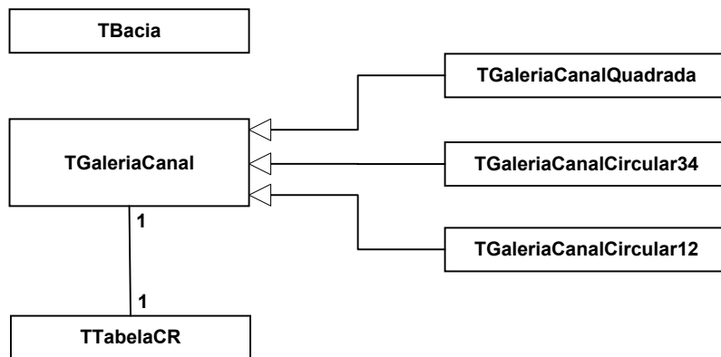
Figura 5 – Classes do problema típico
