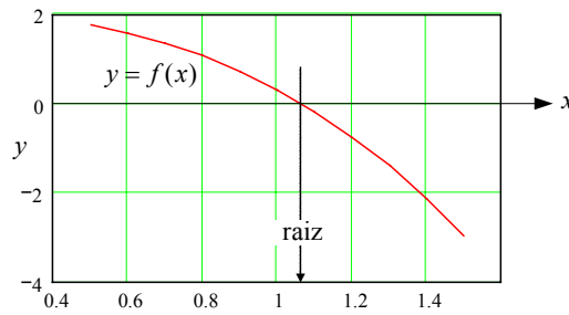
Figura 4 – Raiz da função
