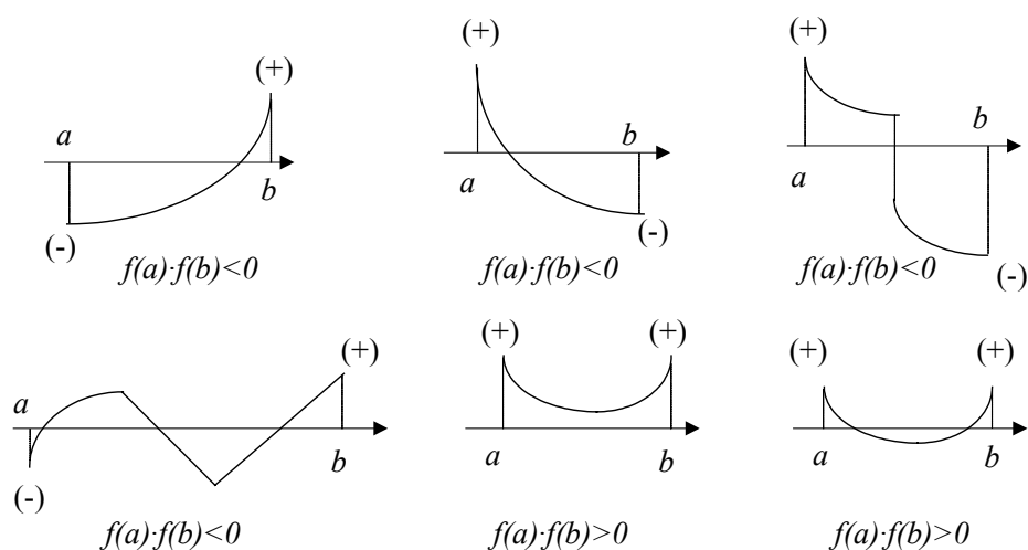
Figura 3 – Ilustrações do Teorema de Bolzano
