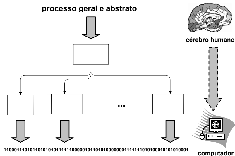
Figura 1 – Domínio da complexidade
