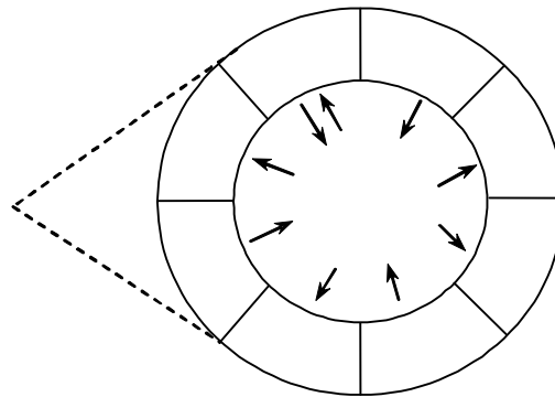
Figura 2 – Funções como módulos de construção
