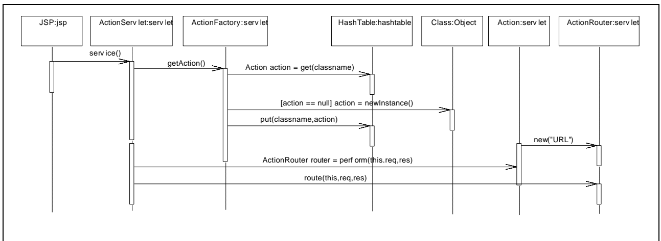
Figura 4: Diagrama de seqüência das servlets responsáveis pelo modelo MVC da aplicação
